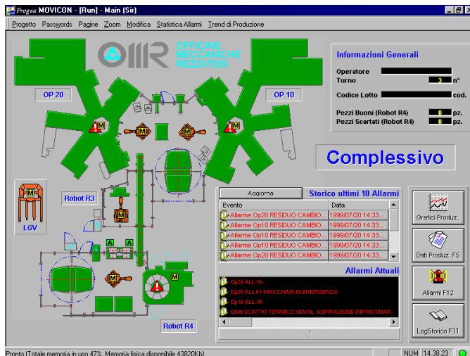
Sinottico principale dell'applicazione di supervisione e analisi dati di produzione realizzata da SIR.
